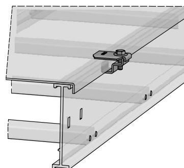
側夾式蓋板夾安裝示意圖
