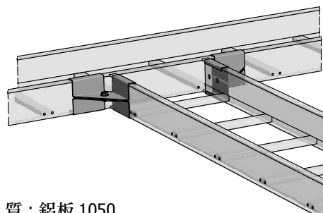
水平側板安裝示意圖
