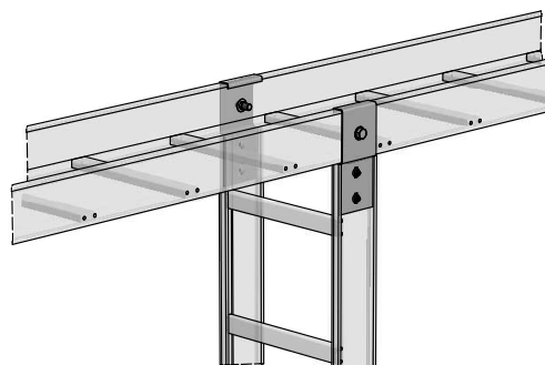
垂直分支板安裝示意圖
