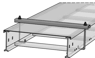
蓋板夾安裝示意圖
