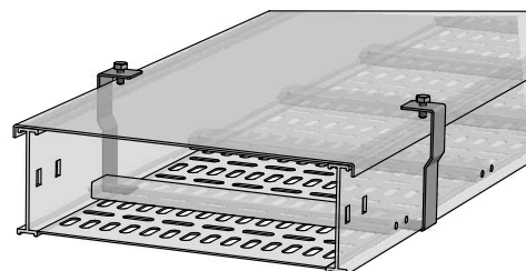
外側式蓋板固定夾安裝示意圖
