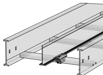
分隔板固定片安裝示意圖
