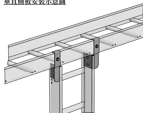
垂直側板安裝示意圖
