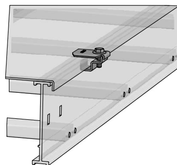
側夾式蓋板夾安裝示意圖
