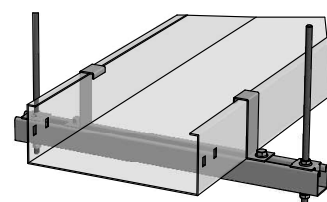
外側固定片安裝示意圖
